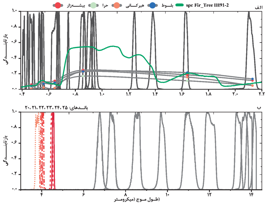
شکل ۳. باندهای طیفی سنجنده مودیس (خطوط خاکستری): محدوده مرئی و فروسرخ میانی و میزان بازتابندگی چهار نوع پوشش جنگلی مهم ایران، همچنین نمونه رفتار طیفی پدیده گیاهی spc Fir_Tree IH91-2 Complete، برگرفته از سایت USGS (الف)؛ محدوده باندهای حرارتی سنجنده مودیس (ب)
