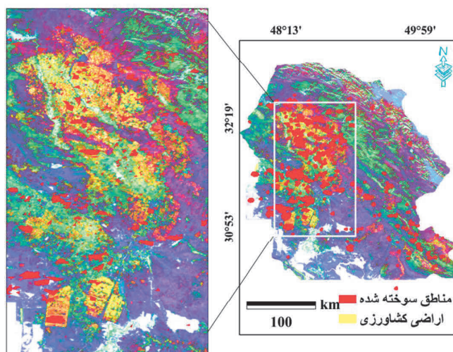
شکل ۷. نقشه تهیه‌شده با استفاده از روش طبقه‌بندی Mahalanobis Distance، از دو شاخص EVI و NDVI سنجنده مودیس در دوم خرداد ۱۳۹۹، استان خوزستان
