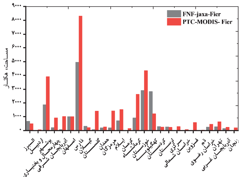
شکل ۹. مقایسه مساحت‌های برآورده‌شده آتش‌سوزی در مناطق جنگلی، براساس نقشه پوشش درصد درخت (PTC) مودیس و نقشه FNF-JAXA
