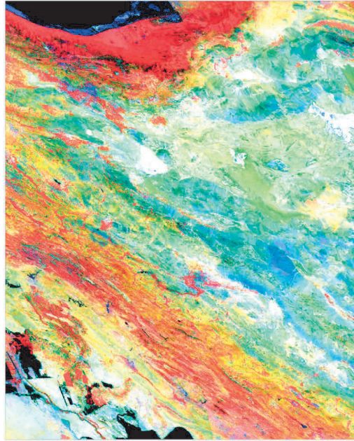
شکل ۲. تصویر ترکیب رنگی کاذب (RGB: NIR, Red, Blue) از باندهای سنجنده مودیس موزاییک h22v05 در کشور ایران (۲۰۲۰/۰۴/۲۱)
