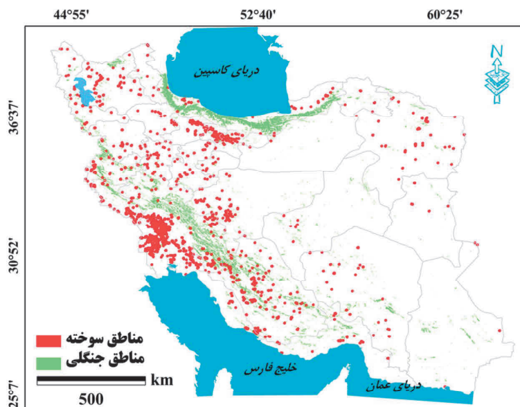
شکل ۵. نقشه ماسک‌شده مناطق آتش‌سوزی با نقشه FNF-JAXA در ایران، بین یازدهم دی ۱۳۹۸ تا هجدهم خرداد ۱۳۹۹ (روزهای ژوئیه ۱۶۰-۱ سال ۲۰۲۰ م).
