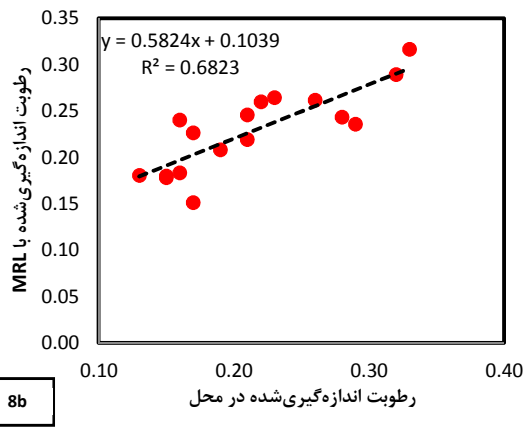
شکل ۸. رابطه بین رطوبت اندازه‌گیری شده با مدل MRL با رطوبت وزنی در \sigma_{HH}^{\circ} : داده آموزشی (a-8) و داده تست (b-8)
