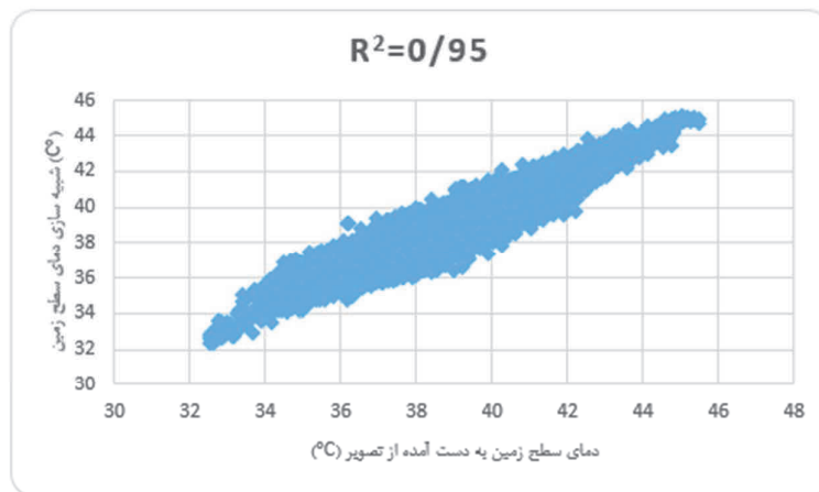
شکل ۹. نمودار پراکنش مقایسه LST در داده واقعی و پیش بینی به منظور ارزیابی دقت
