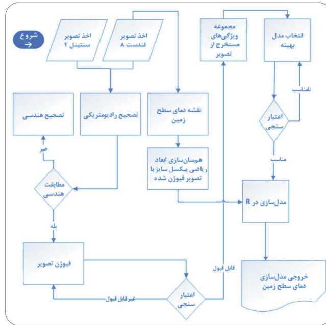
شکل ۳. فلوچارت و مراحل کلی پژوهش
