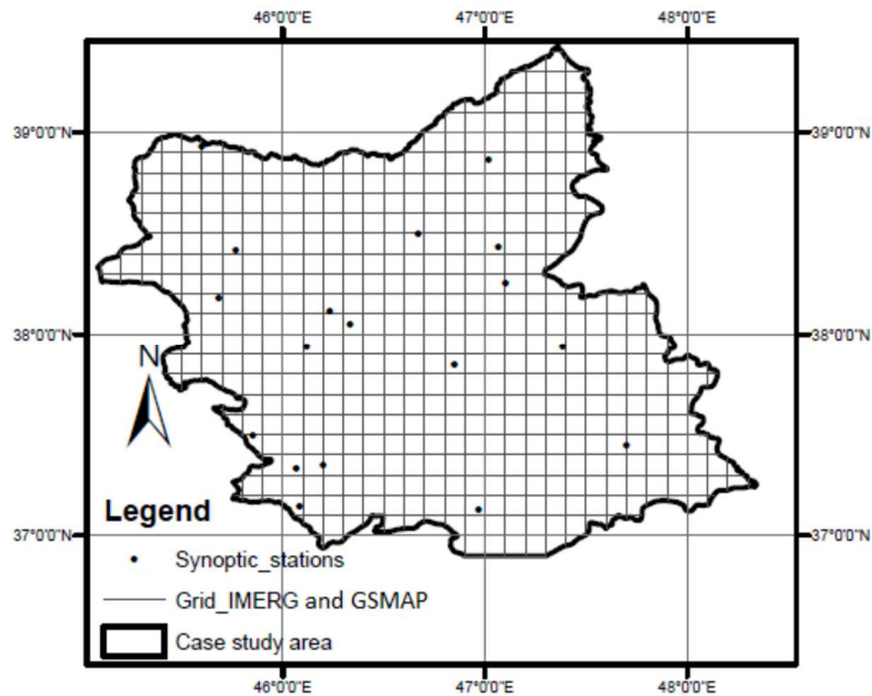
شکل ۲. شبکه سلولی ۰/۱×۰/۱ درجه دوم ماهواره IMERG و GMAP، به همراه موقعیت ایستگاه‌های ثبت بارش زمینی
