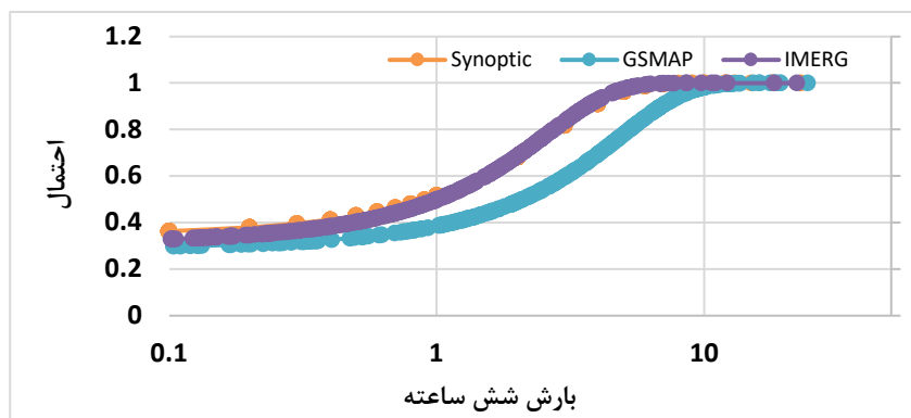
شکل ۶. منحنی احتمال تجمعی و تابع چگالی احتمال داده‌های سینوپتیک، در مقایسه با دو محصول بارشی ماهواره‌ای
