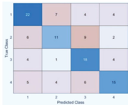
شکل ۷. نتایج به‌دست‌آمده از روش SVM-Adaboost
