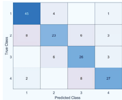
شکل ۵. نتایج به‌دست‌آمده از روش SVM-PSO
