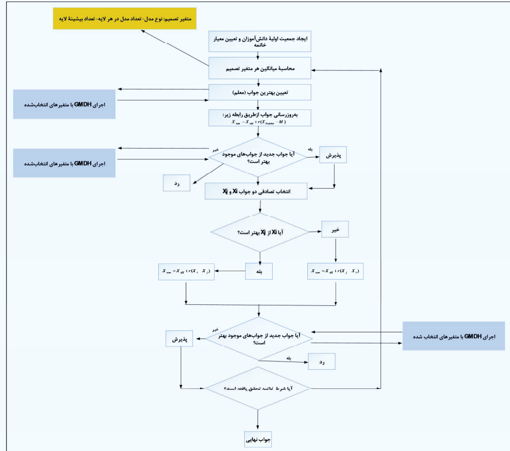
شکل ۱۰. تنظیم پارامترهای شبکه ML-Based GMDH توسعه‌یافته با الگوریتم TLBO
