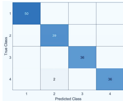
شکل ۹. نتایج حاصل از روش ML-Based GMDH
