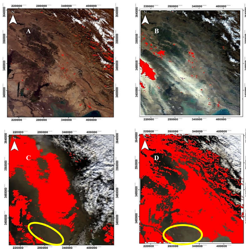
شکل ۸. گردوخاک استخراج‌شده از تصویر MODIS مربوط به هجدهم (A)، نوزدهم (B) بیستم (C) و ۲۱م ژانویه سال ۲۰۱۸ (D) (NDDI)
