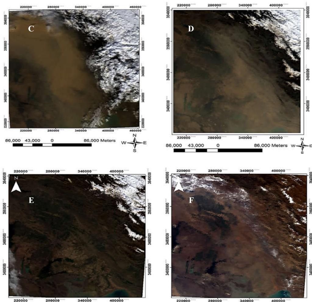
ادامه شکل ۳. تصویر واقعی MODIS در هجدهم ژانویه ۲۰۱۸ (A)، نوزدهم ژانویه ۲۰۱۸ (B)، بیستم ژانویه ۲۰۱۸ (C)، ۲۱م ژانویه ۲۰۱۸ (D)، ۲۶م ژانویه ۲۰۱۹ (E)، ۲۸م اکتبر ۲۰۱۸ (F)
