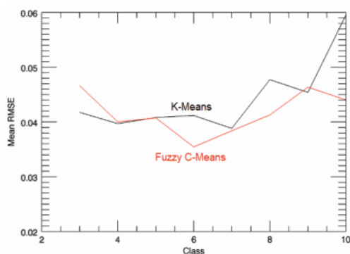
شکل ۱۲. میانگین RMSE برای خوشه‌بندی‌های K-Means و Fuzzy C-Means برای ۱۵ تا ۳ کلاس
