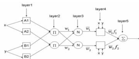
شکل ۳. ساختار ANFIS
