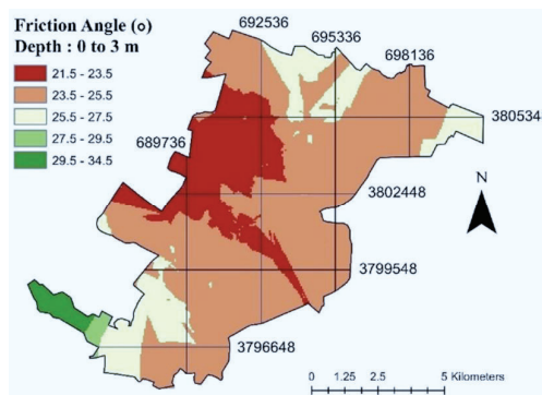
شکل ۵. پهنه‌بندی زاویه اصطکاک (عمق ۰ تا ۳ متر)
