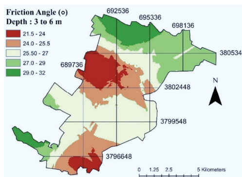
شکل ۶. پهنه‌بندی زاویه اصطکاک (عمق ۳ تا ۶ متر)
