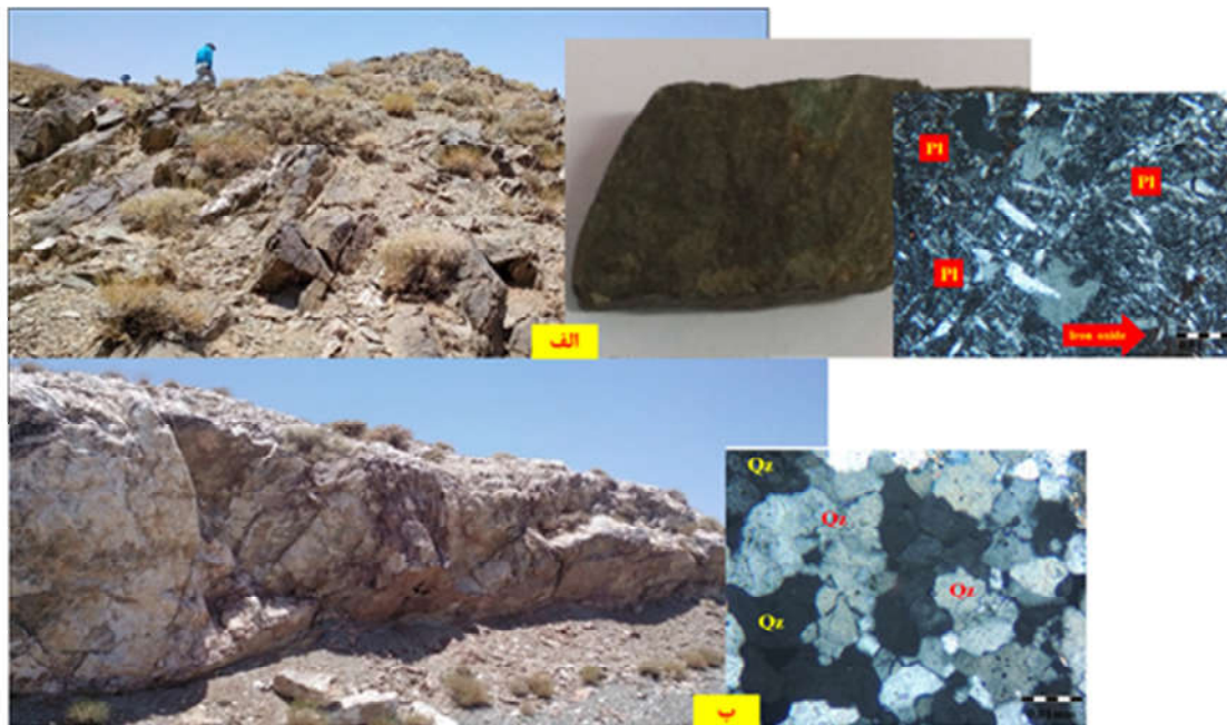
شکل ۳. واحدهای دایک دیابازی (الف)، و کوآرتزیتی در مشاهدات صحرایی به همراه نمونه دستی و مقطع میکروسکوپی آن‌ها (ب).
