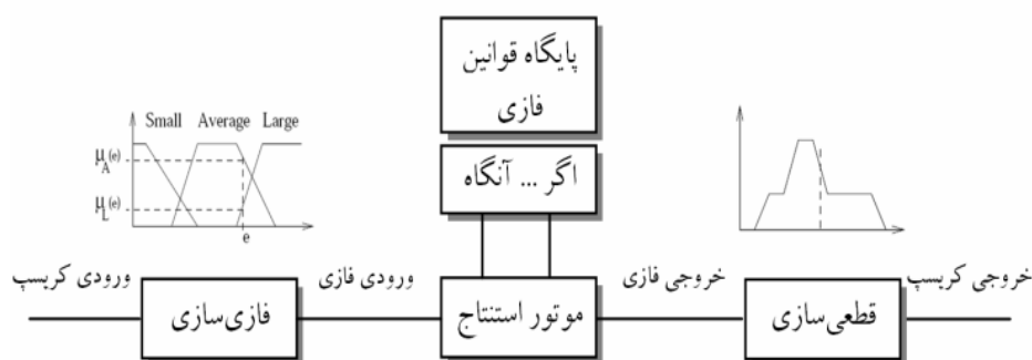
شکل ۱. سیستم استنتاج‌گر فازی منبع: Stefanakis et al., 1996
