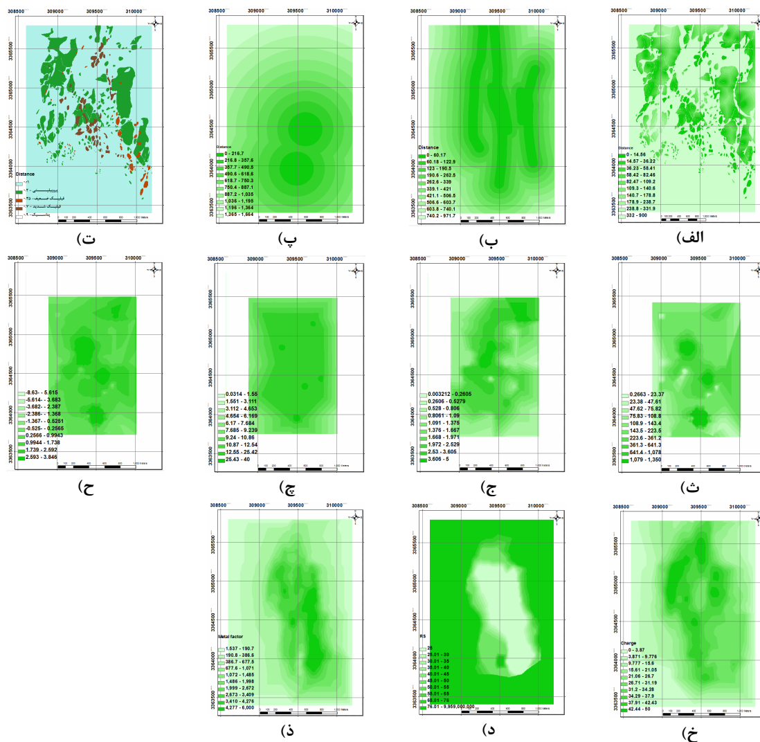
شکل ۶. نقشه فاکتور؛ (الف) وزن منشأ حرارت و سنگ میزبان، (ب) گسل های اصلی، (پ) نشانه های معدنی، (ت) آلتراسیون، (ث) عیار مس، (ج) عیار مولیبدن، (چ) عیار طلا، (ح) ادیتو مس و مولیبدن، (خ) شارژ ابلیت، (د) مقاومت ظاهری، و (ذ) فاکتور فلزی
