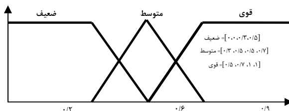
شکل ۲. توابع عضویت فاکتور شارژ ابلیتته
