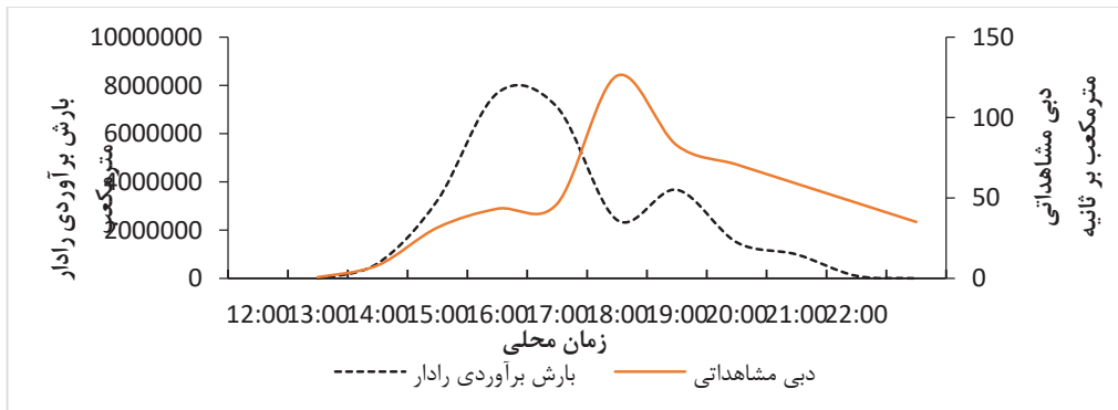
شکل ۶. نمودار دبی و حجم بارش برآوردی رادار برای بارش هشتم خرداد ۱۳۹۳ در حوضهٔ زرین گل
