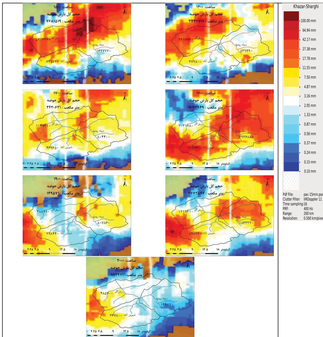
شکل ۷. نمایش پراکنش بارش حوضهٔ زرین گل از ساعت ۱۴:۰۰ تا ۲۰:۰۰، سیل هشتم خرداد ۱۳۹۳
