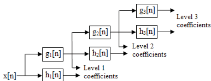
شکل ۲. دیاگرام تبدیل موجک ایستا تا تجزیه سوم (g) فیلتر بالاگذر و h فیلتر پایین گذر است)
