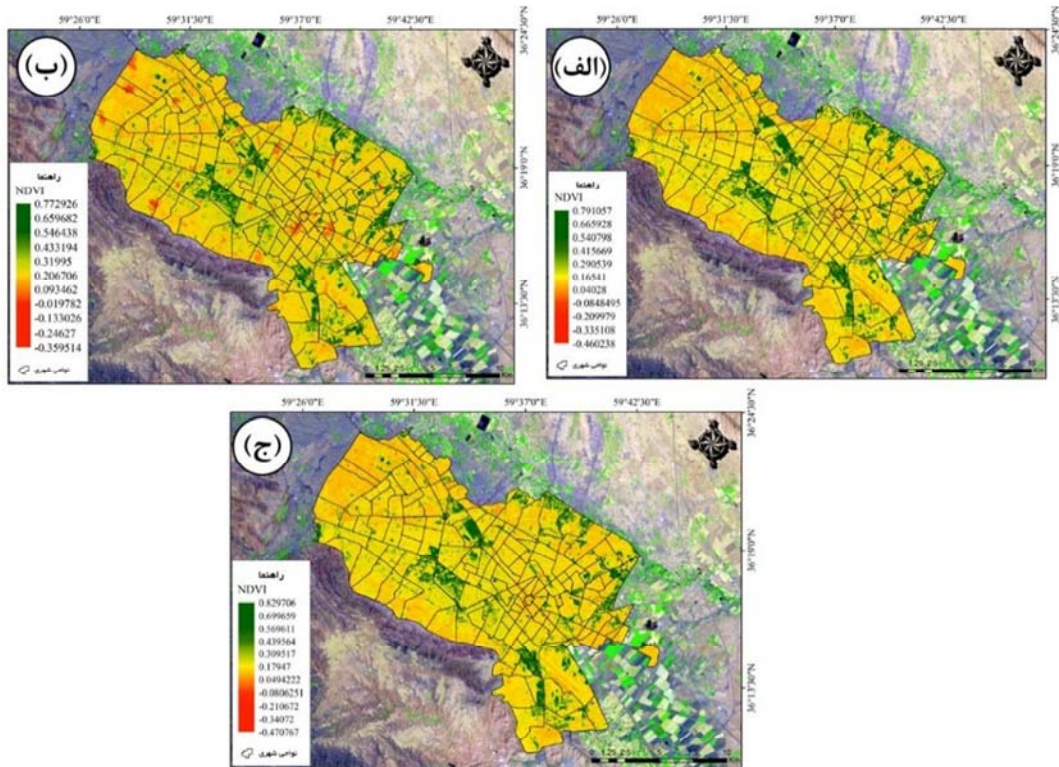
شکل ۶. شاخص تفاضل بهنجار شده پوشش گیاهی (NDVI) مشهد از حسگر OLI ماهواره لندست ۸: (الف) سال ۲۰۱۳؛ (ب) سال ۲۰۱۴؛ (ج) سال ۲۰۱۵
