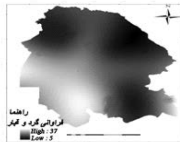
(الف) فراوانی طوفان‌های گرد و غبار
