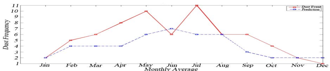
شکل ۲۱. مقدار واقعی و پیش‌بینی‌شده تعداد گرد و غبار برای خاک‌های باتلاقی شور
