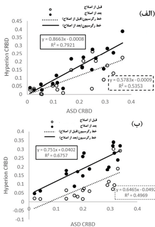
شکل ۱۳. مقایسه CRBD حاصل از به‌کارگیری روش VCCD بر طیف‌های استخراج شده از تصویر هایپریون و طیف‌سنجی آزمایشگاهی؛ برای کانی‌های الف) کائولینیت، ب) مسکویت
