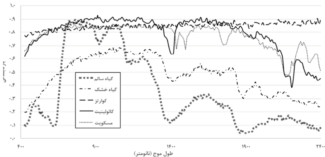
شکل ۷. نمودارهای طیفی شکل ۶ پس از اضافه شدن نویز تصادفی به آنها. نویزها به صورت تصادفی و در بازه ۲۰-۰٪ به طیف‌ها اضافه شدند؛ به گونه‌ای که هر طول موج می‌تواند مقدار متفاوتی از نویز در این بازه را داشته باشد
