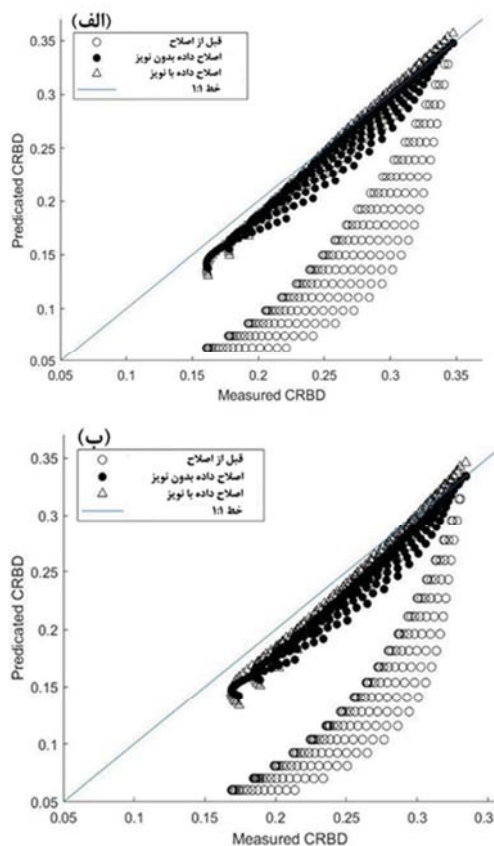
شکل ۱۱. بررسی تأثیر نویز در عملکرد الگوریتم، در برداشتن اثر پوشش گیاهی برای کائولینیت (الف) و مسکویت (ب)
