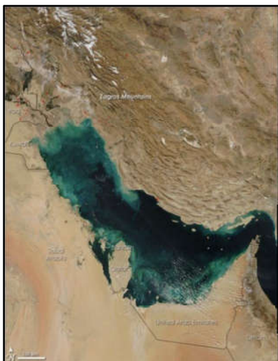
شکل ۲. تصویر ماهواره‌ای خلیج فارس از سنجنده مودیس؛ ۱۳۸۶ آذر ۷
