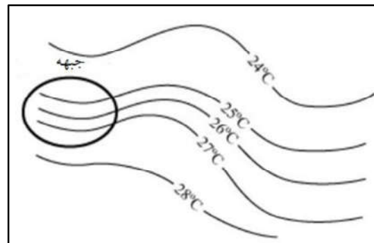
شکل ۴. خطوط همدمای و جبهه دمایی
