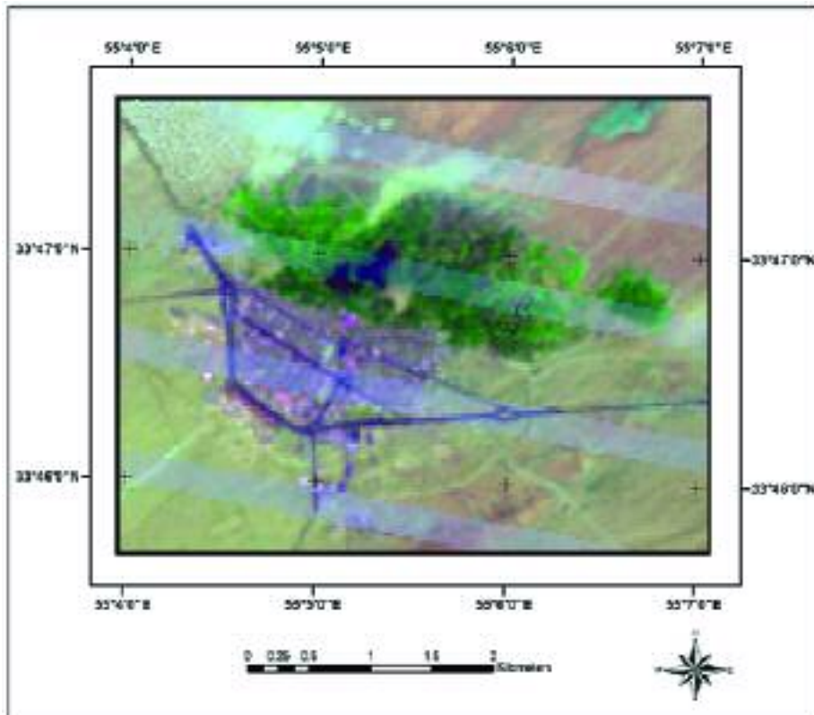
شکل ۹. تصویر ماهواره‌ای لندست منطقه خور پس از آتش‌سوزی
