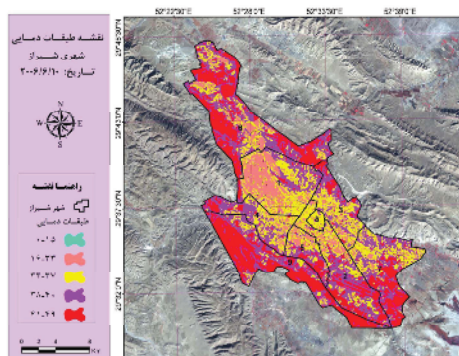
شکل ۵. نقشه طبقه‌بندی دمایی استخراج‌شده از تصویر ماهواره‌ای لندست سنجنده ETM+ شهر شیراز
