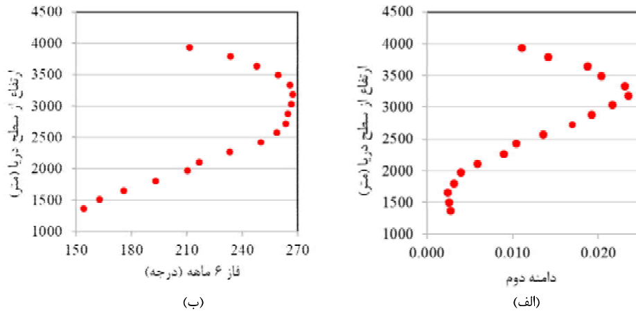
شکل ۱۱. رابطه بین ارتفاع از سطح دریا و دامنه دوم هارمونیک (الف) و نیز ارتفاع از سطح دریا و فاز دوم هارمونیک (ب) براساس سری‌های زمانی ۲۰۱۳، ۲۰۱۴، و ۲۰۱۵
