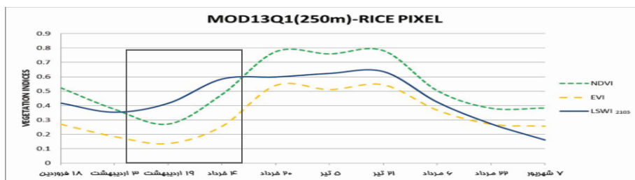
شکل ۲. مقایسه سه شاخص پوشش گیاهی در سال زراعی ۱۳۸۹ در تصاویر MODIS با قدرت تفکیک مکانی ۲۵۰ متر (MOD13Q1) در یک پیکسل برنج (E 28° 24' 42", N 36° 26' 17' 23").
