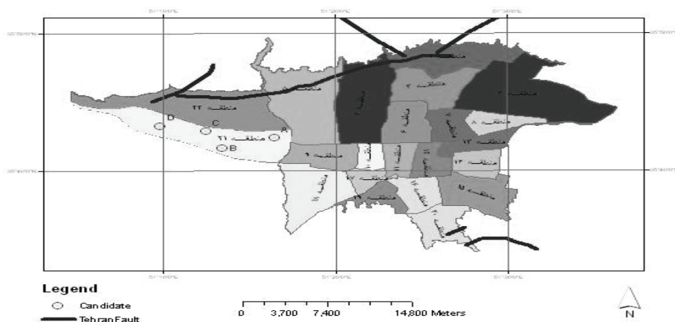
شکل ۷. گسل‌های موجود در شهر تهران
