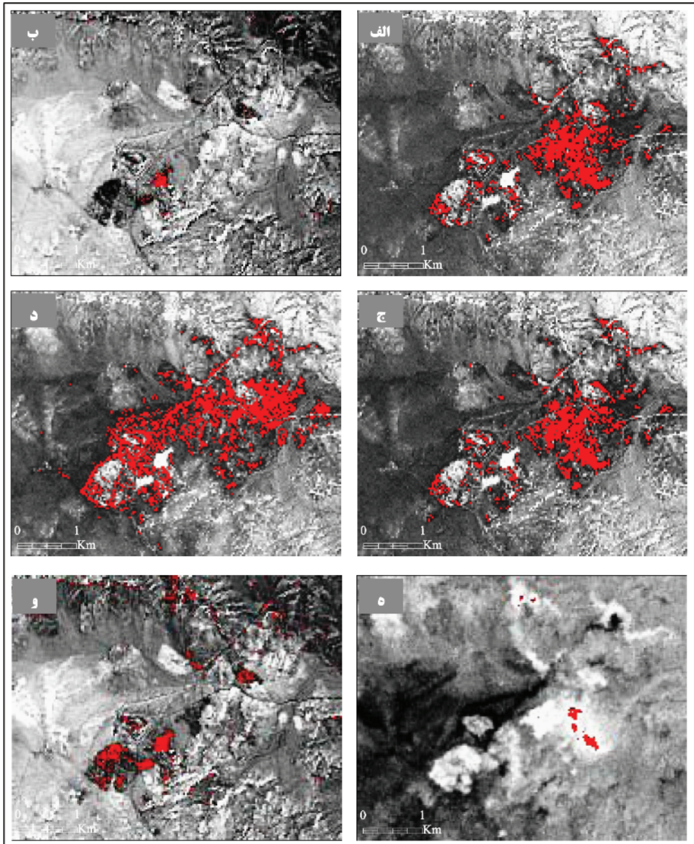
شکل ۸. توزیع مکانی کانی‌های رسی براساس نتایج الگوریتم SAM؛ الف و ب) تصویرهای خروجی SAM نسبت به طیف تصویر کانی‌های کاتولینیت (الف) و پیروفیلیت (ب) به‌دست آمده از روش SMACC؛ ج و د) تصویرهای خروجی SAM نسبت به طیف تصویر کانی‌های کاتولینیت (ج) و پیروفیلیت (د) به‌دست آمده از روش PPI؛ ه، و) تصویرهای خروجی SAM نسبت به طیف کتابخانه‌ای USGS کانی‌های کاتولینیت (ه) و پیروفیلیت (و)
