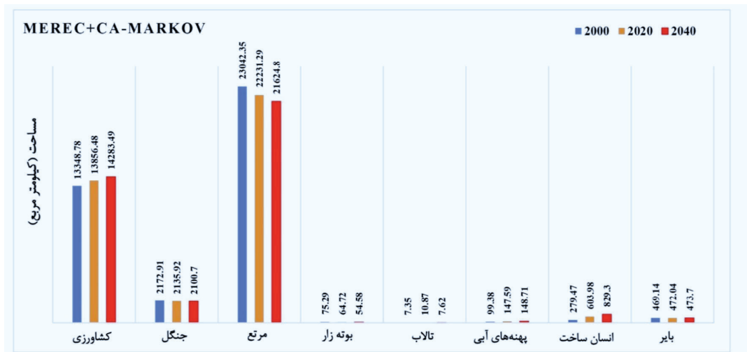
شکل ۸. روند تغییرات LULC در حدفواصل زمانی بین سال‌های ۲۰۲۰ تا ۲۰۴۰ (خروجی مدل MEREC + CA-Markov)
