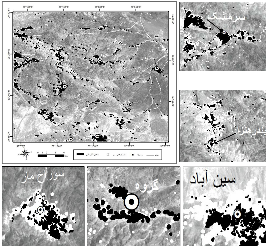
شکل ۲. مناطق استخراج شده با استفاده از روش SAM برای دگرسانی آرژیلیک به رنگ سیاه و فیلیک به رنگ سفید. محدوده کانسارهای موجود در منطقه با بزرگ‌نمایی در اطراف نقشه اصلی نمایش داده شده است.
