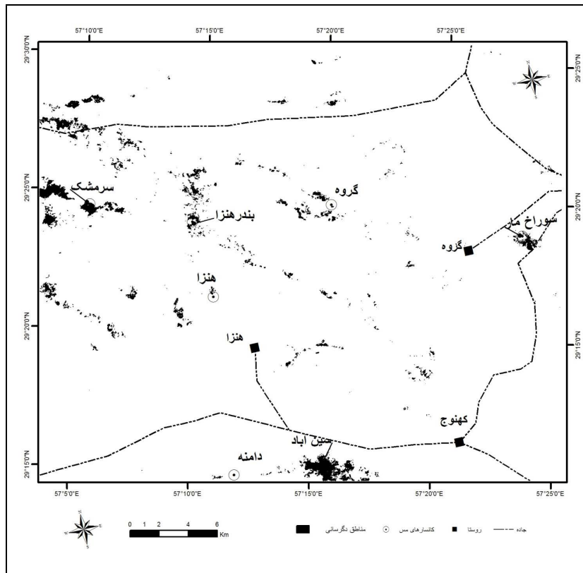
شکل ۴. موقعیت مکانی دگرسانی‌های آرژیلیک و فیلیک را نشان می‌دهد که بیشترین هم‌پوشانی را در دو روش SAM و الگوریتم عملگر منطقی دارند. این مناطق انطباق خوبی با نواحی کانه‌زایی مس پورفیری شناخته شده در منطقه دارند.
