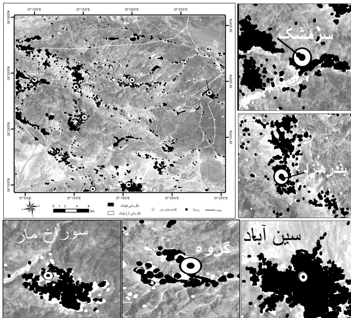
شکل ۳. مناطق استخراج‌شده با استفاده از روش عملگر منطقی برای دگرسانی آرژیلیکی به رنگ سیاه و فیلیک به رنگ سفید مشخص شده است. محدوده کانسارهای موجود در منطقه با بزرگ‌نمایی در اطراف نقشه اصلی نمایش داده شده است.
