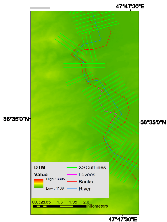
شکل ۶. شمای گرافیکی از نتایج الحاقی HEC GeoRAS
