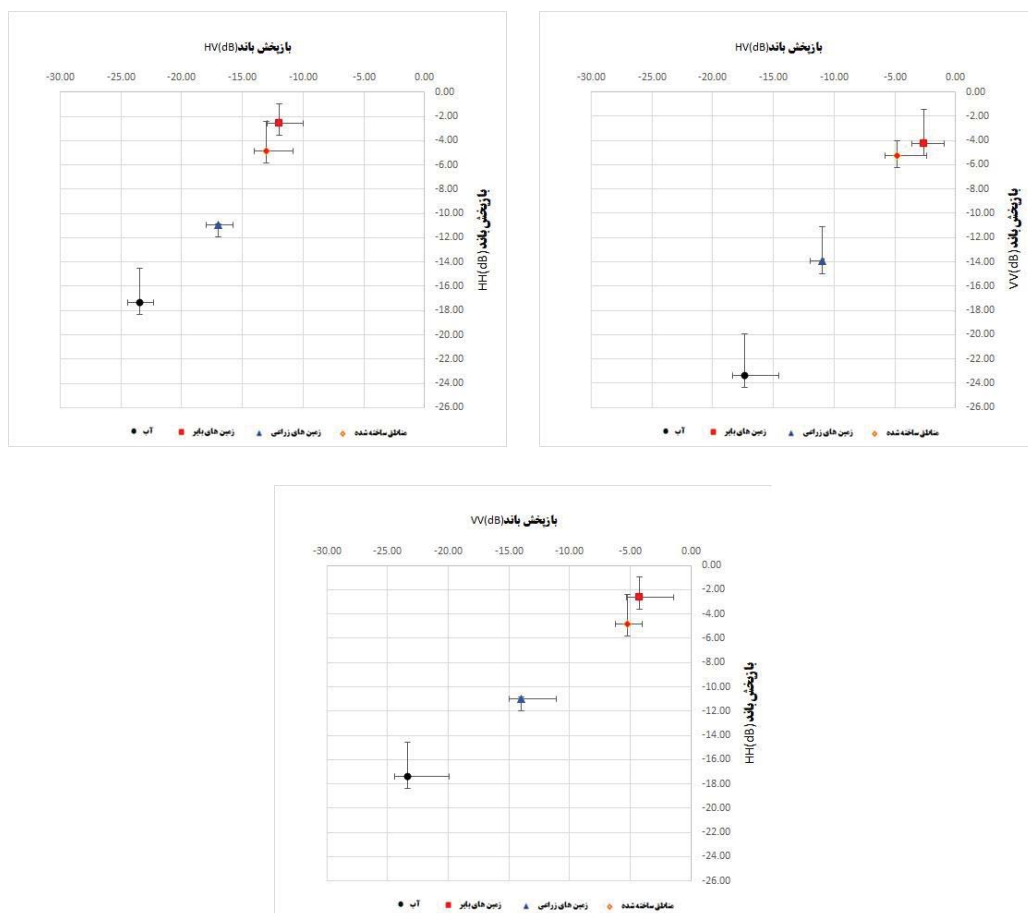
شکل ۱. میانگین و انحراف معیار ضرایب بازیش کلاس‌های متفاوت پوشش زمین در حالت‌های متفاوت دوپولاریمتریک
