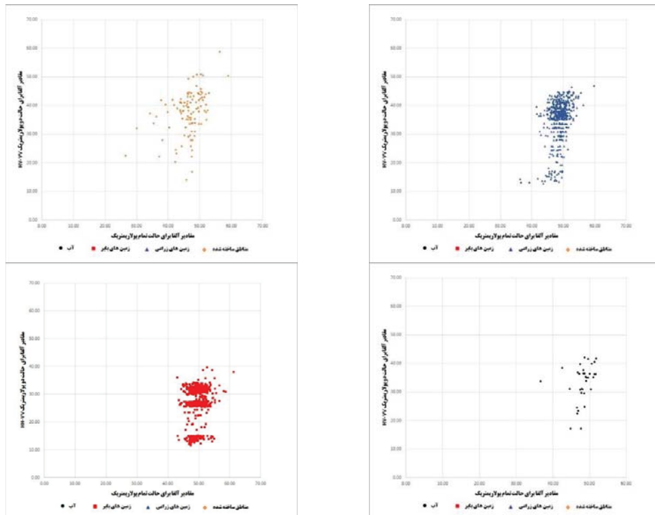
شکل ۴. مقایسه مقادیر آلفا در حالت دوپولاریزمتریک HH-VV، با حالت تمام‌پولاریزمتریک در کلاس‌های متفاوت پوشش زمین
