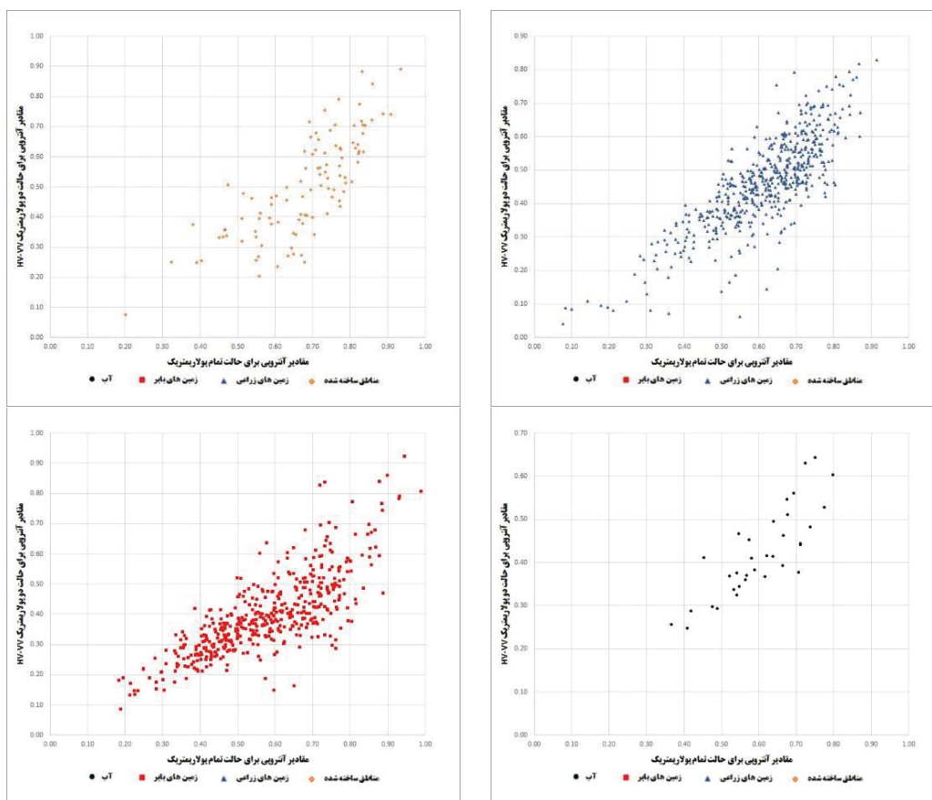
شکل ۷. مقایسه مقادیر آنتروپی در حالت دوپولاریمتریک HV-VV با حالت تمامپولاریمتریک، در کلاس‌های متفاوت پوشش زمین
