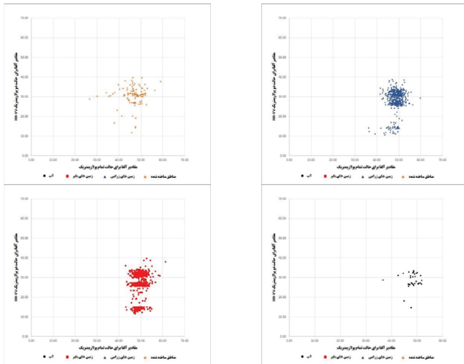
شکل ۳. مقایسه مقادیر آلفا در حالت دوپولاریزمتریک HH-VV با حالت تمام‌پولاریزمتریک در کلاس‌های متفاوت پوشش زمین
