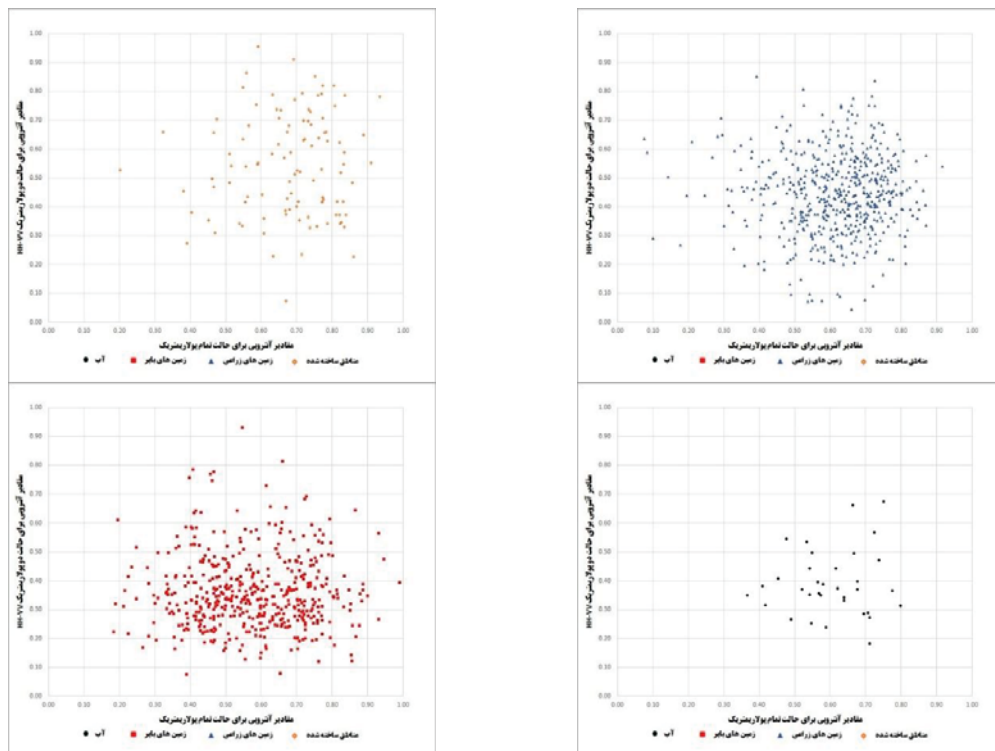
شکل ۶. مقایسه مقادیر انترویی دوپولاریمتریک HH-VV با تمامپولاریمتریک، در کلاس‌های متفاوت پوشش زمین
