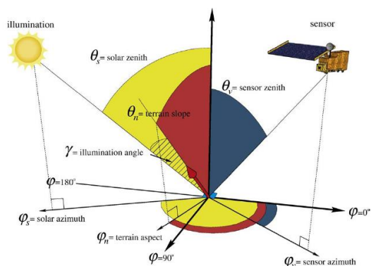
شکل ۷. (a) منحنی میزان پیکسل نمونه، (b) نمای شماتیک موقعیت سنجنده و خورشید نسبت به پیکسل برای ایجاد برق خورشیدی منبع: برگرفته از Sirguy et al., 2009
