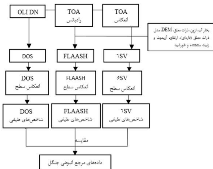
شکل ۳. نمودار جریان تصحیح اتمسفریک لندست ۸ با استفاده از مدل‌های DOS، FLAASH و 6SV.
