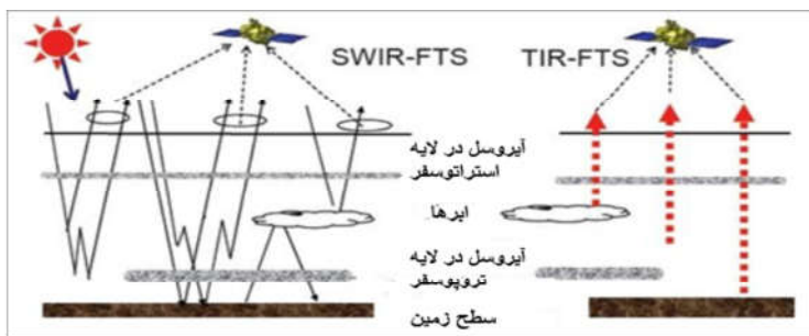
شکل ۱. انتقال‌های تابشی SWIR-TIR در جو زمین
