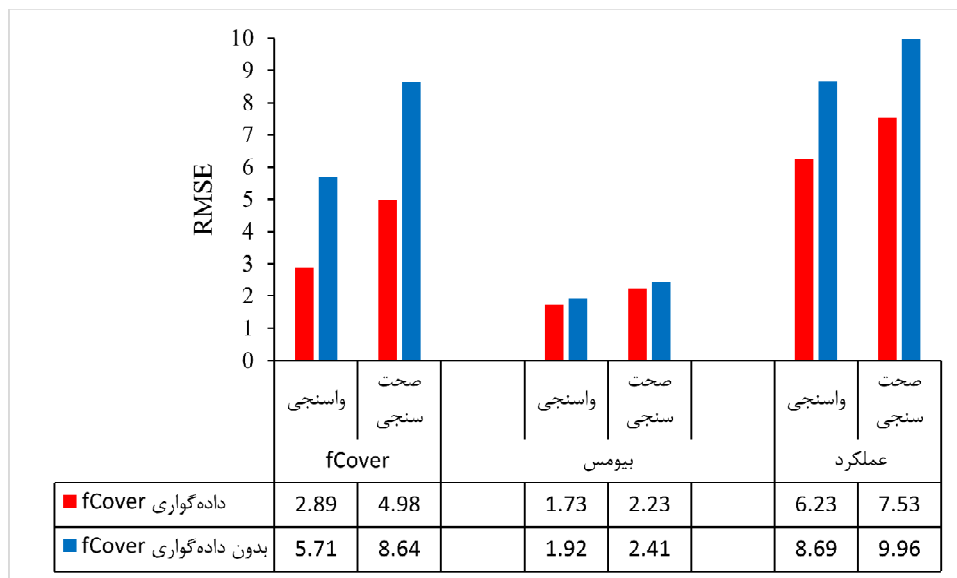
شکل ۴. ارزیابی نتایج مدل AquaCrop. RMSE در متغیرهای خروجی fCover، بیومس و عملکرد علوفه‌ای، به‌ترتیب برحسب درصد، ton/ha و ton/ha است. (fCover و بیومس در کل دوره رشد گیاه با ۶۰ نمونه واسنجی، ۱۲۰ نمونه صحت‌سنجی)، عملکرد (علوفه‌ای) (درانتهای دوره رشد گیاه با ده نمونه واسنجی و بیست نمونه صحت‌سنجی))
