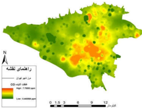
شکل ۸. توزیع مکانی غلظت آلاینده CO مدل LUR کلی، در تابستان ۱۳۹۶ سنجش از دور و GIS ایران سال دوازدهم = شماره اول = بهار ۱۳۹۹
