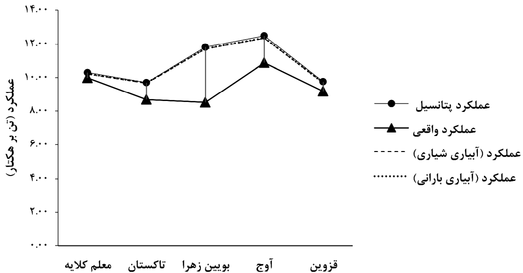
شکل ۵. نمودار عملکرد واقعی و پتانسیل و شکاف عملکرد
