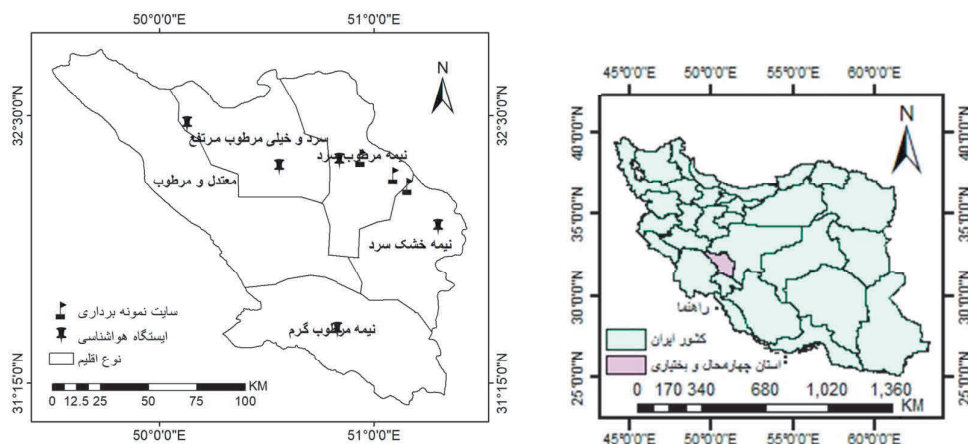
شکل ۱. موقعیت جغرافیایی استان چهارمحال و بختیاری در ایران و اقلیم‌های منطقه مطالعاتی، همراه با ایستگاه‌های هواشناسی و سایت‌های نمونه‌برداری
