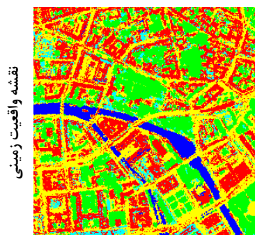
سنجنده: HyMap ابعاد پیکسل: ۲,۵ متر محدوده طیفی: ۲,۵-۴۵,۰ میکرومتر تعداد باندهای طیفی: ۱۱۴ ابعاد: ۳۰۰×۳۰۰ پیکسل
