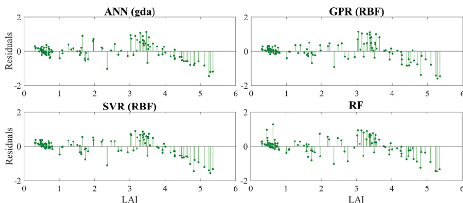
شکل ۳. میزان انحراف مقادیر LAI بازیابی‌شده از مقادیر اندازه‌گیری‌شدهٔ زمینی به‌نسبت خط ۱-۱
