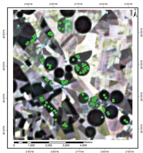
شکل ۱. تصویر ماهواره‌ای کریس- پروبا (ترکیب باندی ۸-۱۲-۲۵ RGB) از منطقه باراکس اسپانیا و پراکنش نمونه‌های برداشت‌شده زمینی LAI (نقاط سبز)
