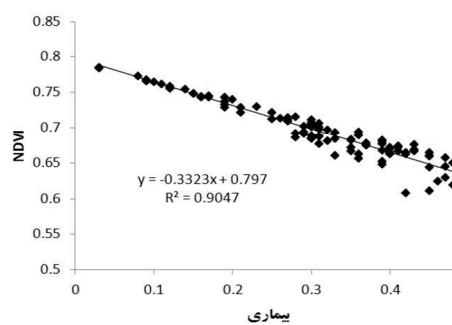
شکل ۵. رابطه شاخص NDVI با افزایش نسبت بیماری از سالم تا ۵۰٪ برگ (سمت چپ) و ۵۰٪ برگ تا ۱۰۰٪ (سمت راست)
