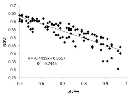
شکل ۵. رابطه شاخص NDVI با افزایش نسبت بیماری از سالم تا ۵۰٪ برگ (سمت چپ) و ۵۰٪ برگ تا ۱۰۰٪ (سمت راست)
