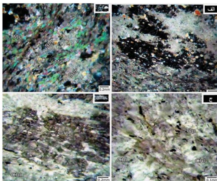
شکل ۳. مقطع میکروسکوپی نمونه ب محدوده مورد مطالعه: در برداری کوارتز در بلور پورفیروبلست گارنت (حاوی انکلوژیون‌های کوارتز) در زمینه سربیتی (الف)؛ بلورهای موسکویت و سربیت جهت یافته (ب)؛ نور PPL نشان‌دهنده کانه‌های مات در زمینه کلریتی (ج)؛ نمایی از بلورهای پورفیروبلست گارنت در نور PPL که کم‌وبیش با کلریت جانشین شده است.
