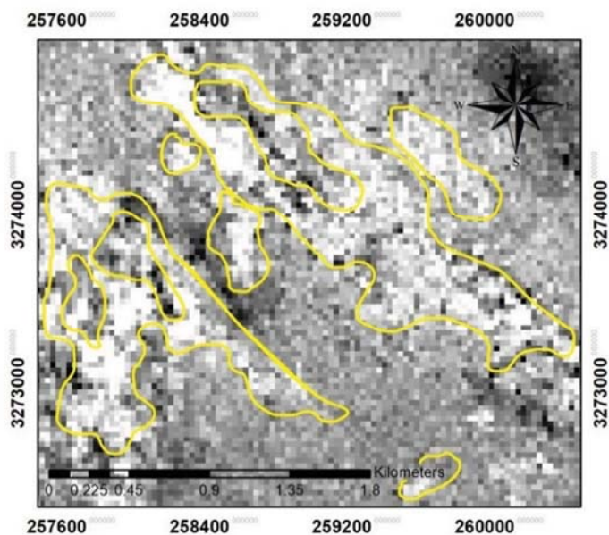
شکل ۷. نسبت‌گیری باندهی (B5+B7)/B6 و آنومالی‌های آلتراسیون فیلک (کانن‌زایی آهن‌دار) در منطقه مورد مطالعه (مناطق روشن در شکل نشان‌دهنده مناطق کانن‌زایی آهن‌دار و آلتراسیون فیلک در منطقه مورد مطالعه است که دارای روند عمومی شمال‌غرب-جنوب‌شرق‌اند)
