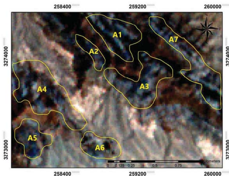
شکل ۴. ترکیب رنگی (۱۲۳) RGB و آنومالی های کانی زایی آهن دار با رنگ آبی تیره، در منطقه مورد مطالعه (آنومالی های A1، A2، A3، A7 و در نیمه شمالی محدوده و آنومالی های A4، A5 و A6 در نیمه جنوبی محدوده واقع شده است که موازی یکدیگر و منطبق بر روند ساختارهای زمین شناسی منطقه اند)
