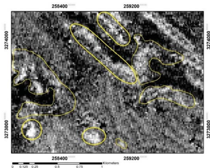
شکل ۶. نسبت‌گیری باندهی Band 5 / Band 4 و آنومالی‌های کانن‌زایی آهن‌دار در منطقه مورد مطالعه
